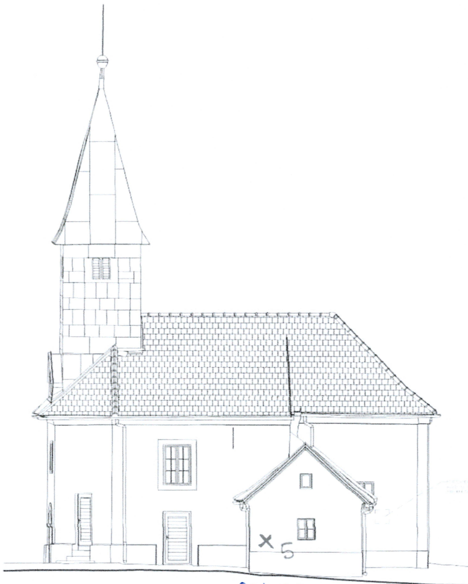
JUŽNO PROČELJE
