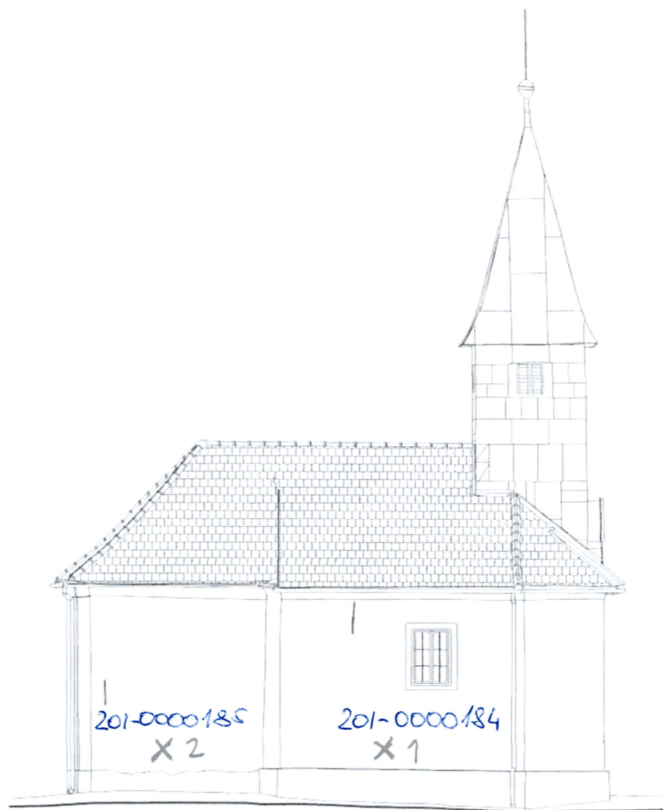
SJEVERNO PROČELJE
